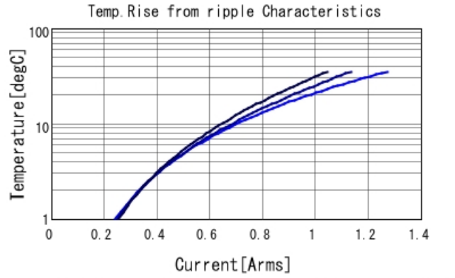
GRM1555C1H750JA01 Temp. rise — 200MHz — 500
