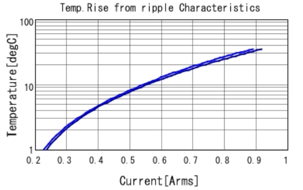
GQM2195G2E1R2CB12 Temp. rise — 2GHz — 3GHz
