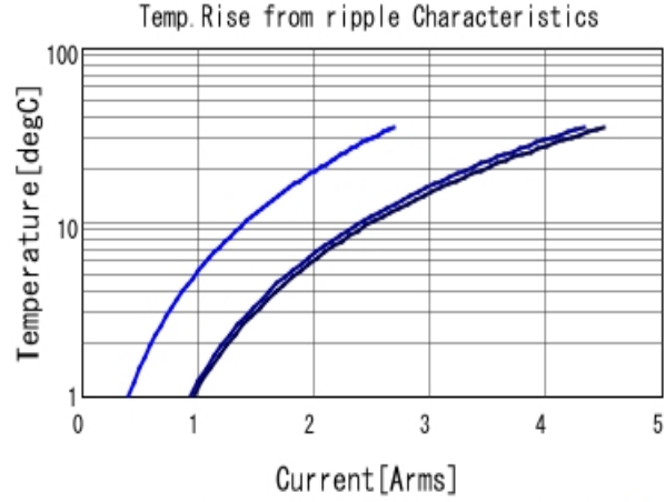
GRM188C70J225KE20 Temp. rise ■ 100kHz ■ 500kHz ■ 1MHz
