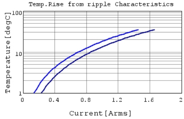
GRT033R61A224KE01 Temp.rise — 600kHz
