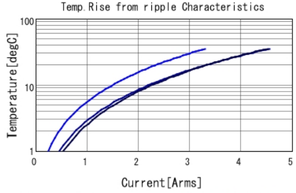
GRM188D71A106KA73 Temp. rise ■ 80kHz ■ 400kHz ■ 800kHz
