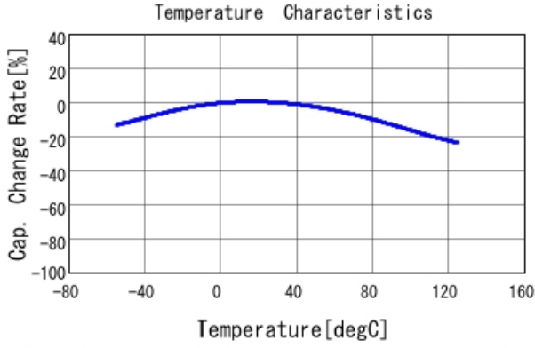
■ GRM188D71A106KA73 C-Temp. capchange, DCO. 0V, ACO. 2Vrm
