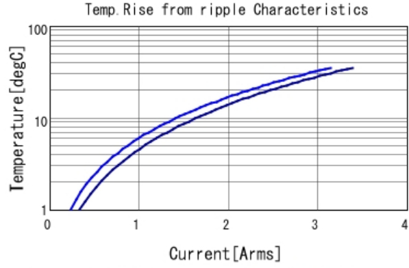
GCH188C71A225KE01 Temp. rise 500kHz 1MHz
