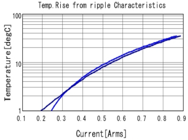
GQM2195C2E1R6CB12 Temp. rise ■ 2GHz ■ 3GHz
