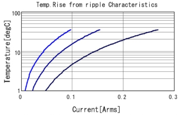
GRJ21AR72E472KWJ1 Temp. rise — 30kHz — 100kHz
