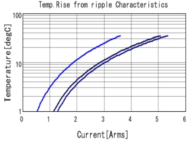
■ GRT31CR61E106KE01 Temp. rise ■ 80kHz ■ 400kHz ■ 800kHz
