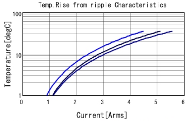
GRM31CD71H106KE11 Temp. rise ■ 80kHz ■ 400kHz ■ 800kHz
