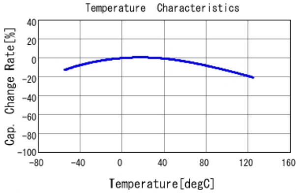
■ GRM31CD71H106KE11 C-Temp. capchange, DCO. 0V, ACO. 1V rm
