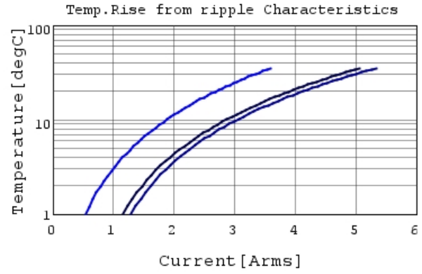
GRT31CC81E106KE01 Temp.rise — 80kHz
