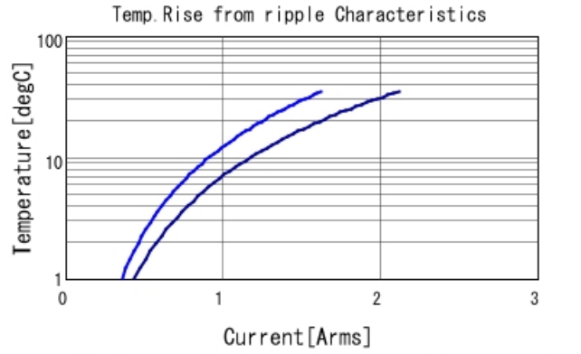
GRM31MR72A154KA01 Temp. rise — 500kHz — 1MHz
