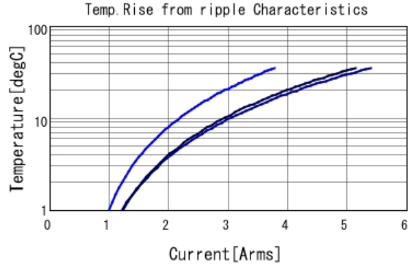
GRM32ER72A225MA35 Temp. rise — 100kHz — 500
