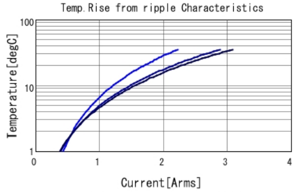
GCJ31CR71H684KA01 Temp. rise — 200kHz — 500
