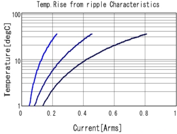
GCJ32DR72J333KXJ1 Temp. rise ■ 30kHz ■ 100kHz ■ 300kHz
