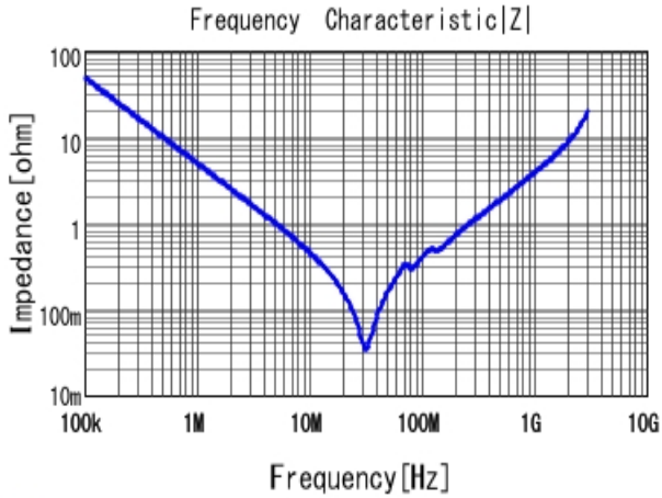
■ GCJ32DR72J333KXJ1 |Z| DC0V, 25degC
