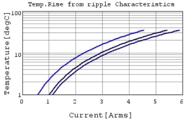
GRT31CC81C226KE01 Temp.rise — 80kHz —
