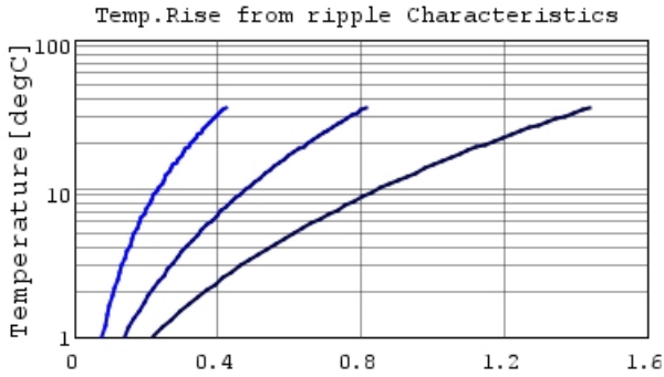
GR332DD72J333KW01 Temp.rise — 30kHz —
