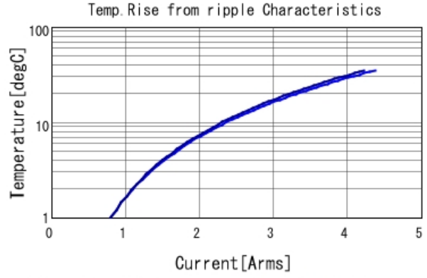
GRM188C81E475KE11 Temp. rise ■ 500kHz ■ 1MHz
