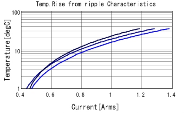
GJM1555C1H300FB01 Temp. rise — 500MHz — 700I
