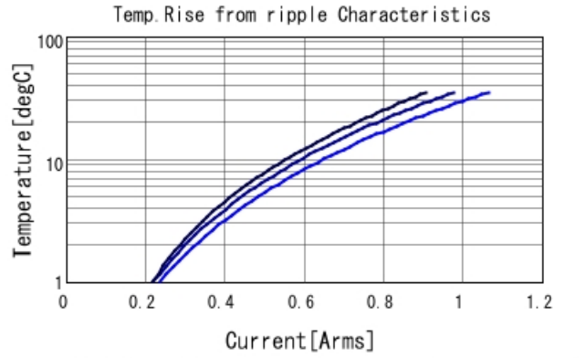
GRM1555C1H180GA01 Temp. rise — 500MHz — 700I
