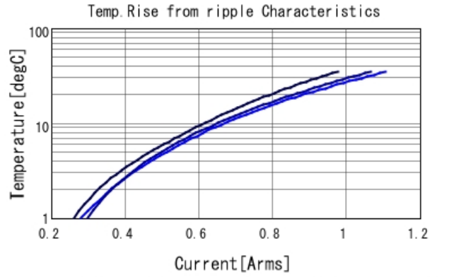
GJM1555C1H120JB01 Temp. rise — 700MHz — 1GHz
