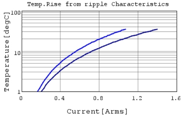
GRT155R71H104KE01 Temp.rise — 500kHz —
