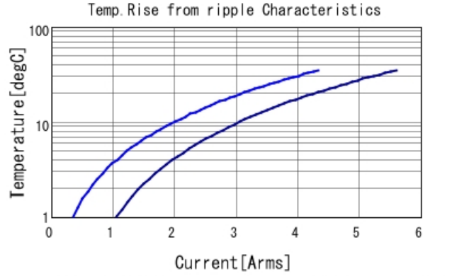
GRM219R61E106KA12 Temp. rise — 100kHz — 500
