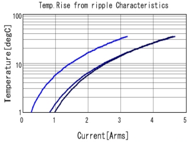
GRT188C80J475ME01 Temp. rise ■ 100kHz ■ 500kHz ■ 1MHz
