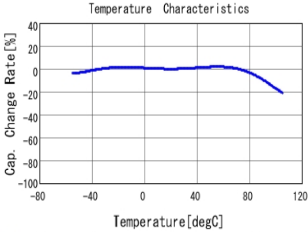
GRT188C80J475ME01 C-Temp. capchange, DCO. 0V, ACO. 5Vrm
