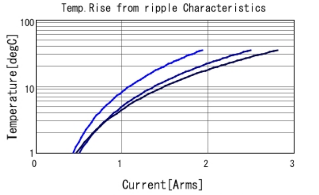
GCJ21BR71E334MA01 Temp. rise — 300kHz — 600
