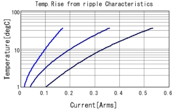
GRJ21BR72E223KWJ3 Temp. rise — 30kHz — 100kHz
