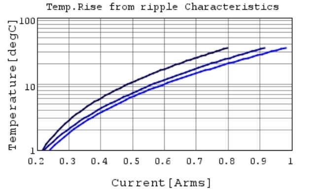
GRT1555C1H6R0DA02 Temp.rise — 700MHz —
