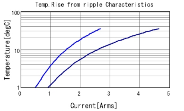
GRM55RR71H105KA01 Temp. rise — 100kHz — 1MHz
