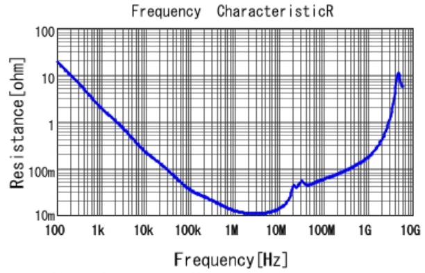
GCJ21BR71E394KA01 R DCOV, 25degC
