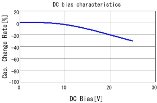
GCJ21BR71E394KA01 C-DC bias capchange, 25.0degC, A
