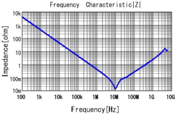
GCJ21BR71E394KA01 |Z| DCOV, 25degC
