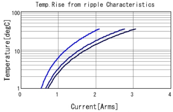
GCJ21BR71E394KA01 Temp. rise — 300kHz — 600
