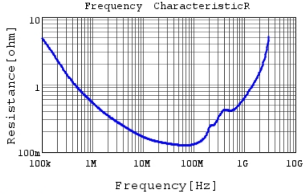
GCJ31BR73A472KXJ1 R DC0V, 25degC
