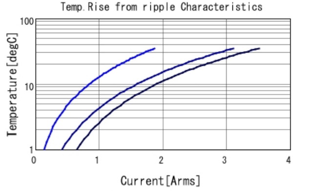
GRM316D71C225KA12 Temp. rise — 100kHz — 500
