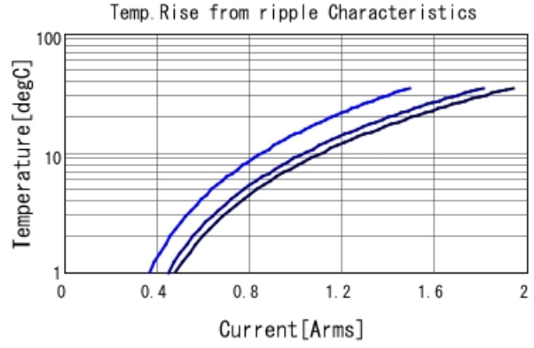
GRM188R71A334KA61 Temp. rise — 300kHz — 600
