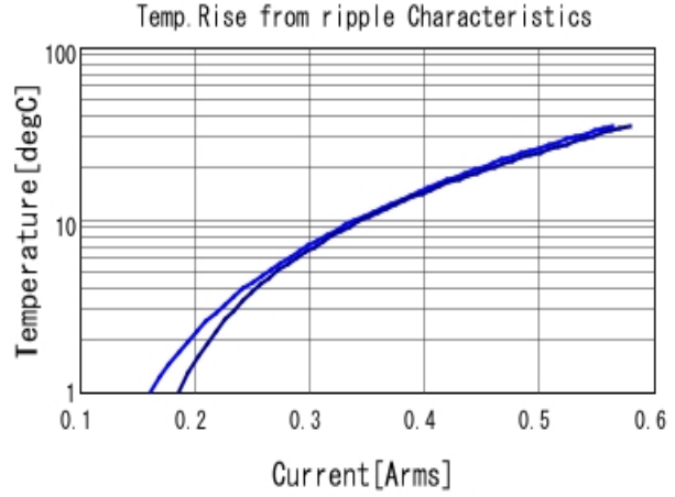
■ GQM22M5C2H1R3BB01 Temp. rise ■ 2GHz ■ 3GHz
