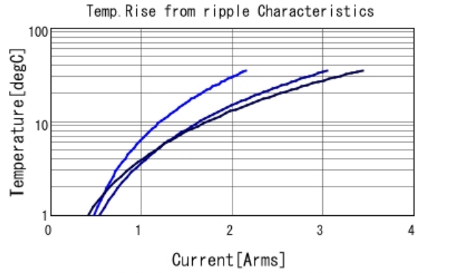
GCJ31CL8YA564KA01 Temp. rise — 200kHz — 500
