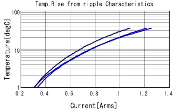
GJM1555C1H180JB01 Temp. rise — 700MHz — 1GHz
