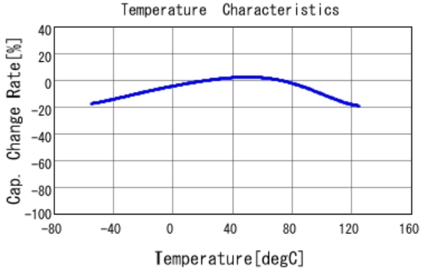
■ GRM21BC71E475KE11 C-Temp. capchange, DCO. 0V, ACO. 5Vrm
