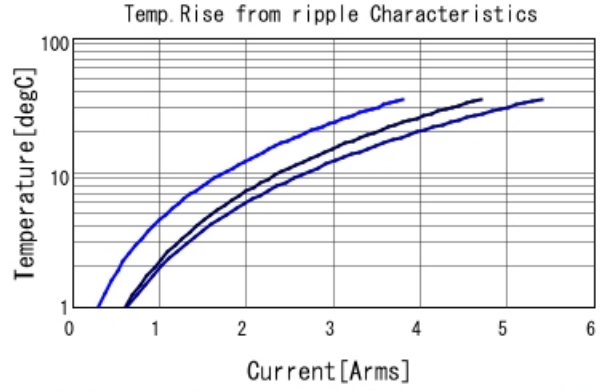
GRM21BC71E475KE11 Temp. rise ■ 100kHz ■ 500kHz ■ 1MHz
