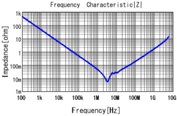
■ GRM21BC71E475KE11 |Z| DCOV, 25degC
