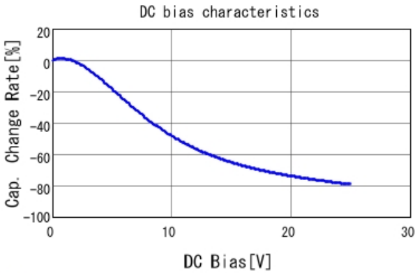
■ GRM21BC71E475KE11 C-DC bias capchange, 25.0degC, AC1V
