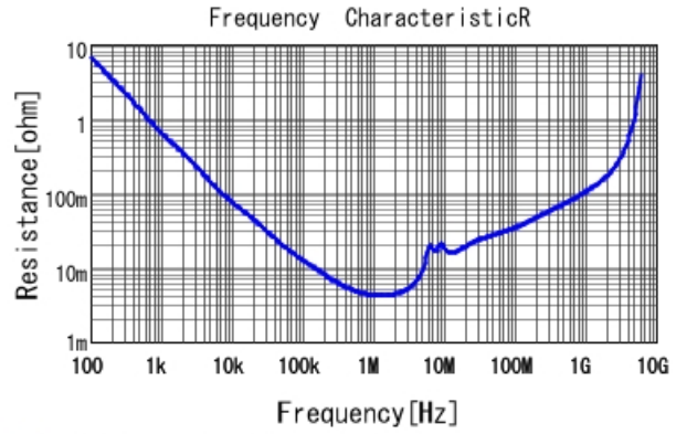
■ GRM21BC71E475KE11 R DCOV, 25degC
