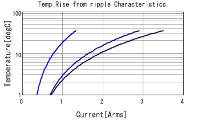
GRM21BR71C474MA01 Temp. rise — 100kHz — 500
