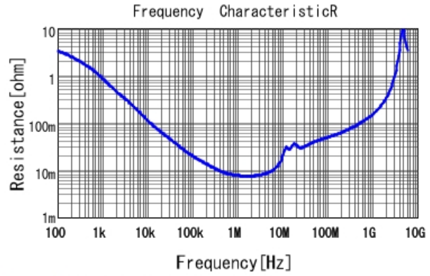
GCJ21BR71C105MA01 R DCOV, 25degC
