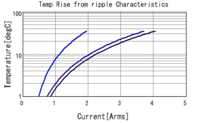
GCJ21BR71C105MA01 Temp. rise — 100kHz — 500
