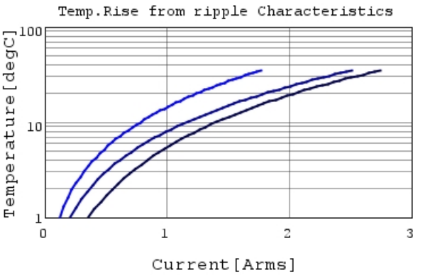
GCJ188R70J225KE01 Temp.rise 100kHz
