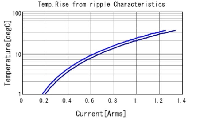
GCM155R71H104KE02 Temp. rise — 800kHz — 1MHz
