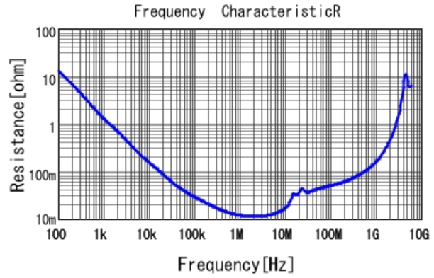
GCJ21BR71E684KA12 R DCOV, 25degC
