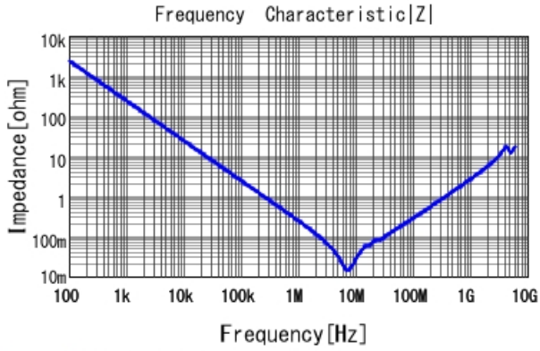
GCJ21BR71E684KA12 |Z| DCOV, 25degC
