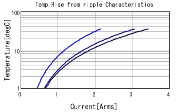
GCJ21BR71E684KA12 Temp. rise — 200kHz — 500
