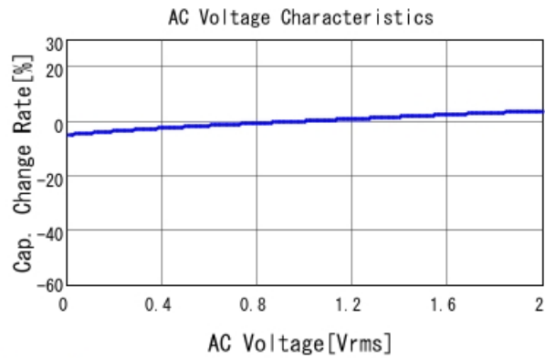
GCJ21BR71E684KA12 C-AC Voltage capchange, DCOV, 25
