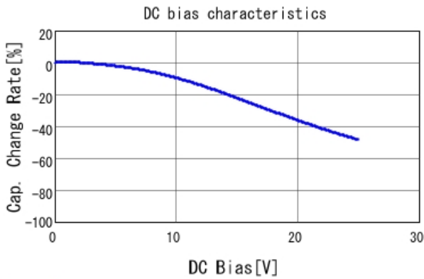
GCJ21BR71E684KA12 C-DC bias capchange, 25.0degC, A
