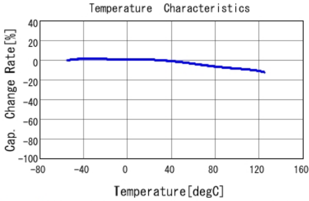
GCJ21BR71E684KA12 C-Temp. capchange, DC0.0V, AC1.C
