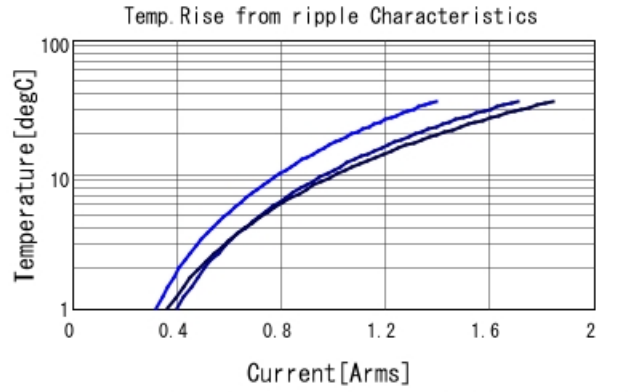
GCJ21BL8YA224KA01 Temp. rise — 300kHz — 600
