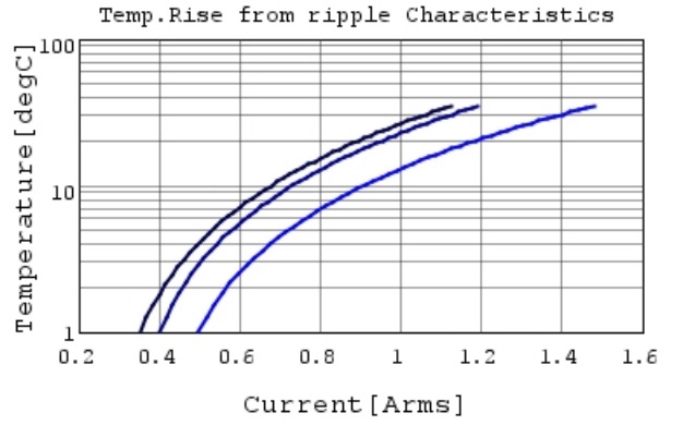
GJM0335C1E150JB01 Temp.rise 400MHz
