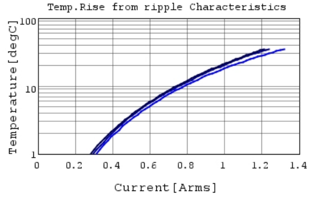
GQM1875C2E180GB12 Temp.rise 500MHz
