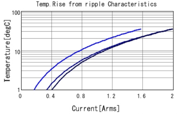
GCM188R71H154KA64 Temp. rise — 400kHz — 800
