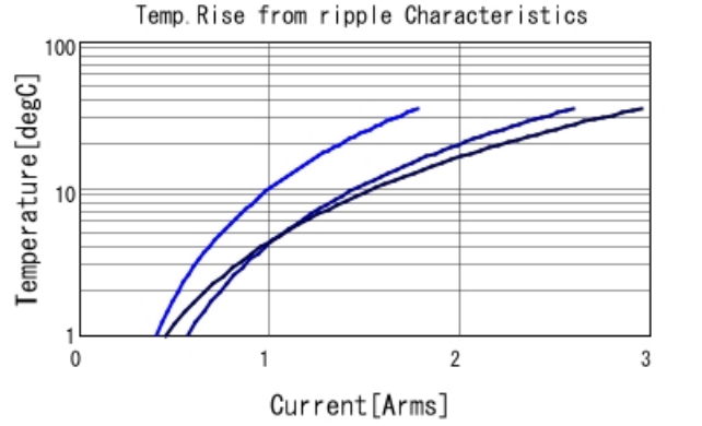
GCJ219R71E474KA12 Temp. rise — 200kHz — 500
