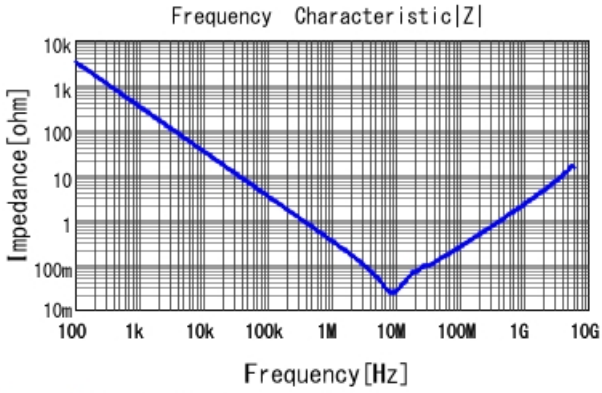
GCJ219R71E474KA12 |Z| DCOV, 25degC
