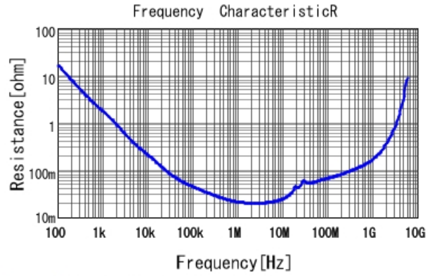
GCJ219R71E474KA12 R DCOV, 25degC
