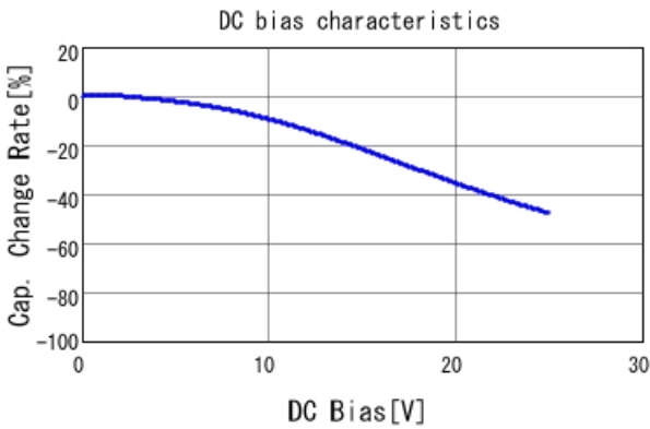
GCJ219R71E474KA12 C-DC bias capchange, 25.0degC, A
