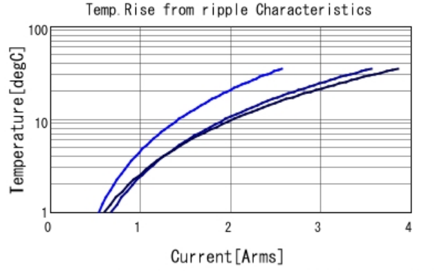
GCJ31CL8YA824KA01 Temp. rise — 200kHz — 500
