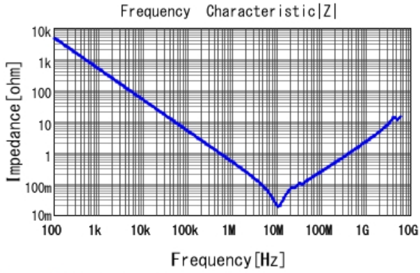
GCJ21BR71E334KA01 |Z| DCOV, 25degC
