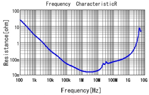
GCJ21BR71E334KA01 R DCOV, 25degC
