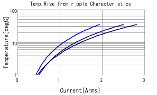
GCJ21BR71E334KA01 Temp. rise — 300kHz — 600
