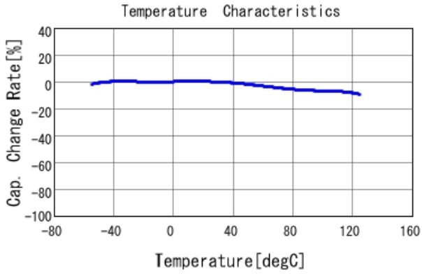
GCJ21BR71E334KA01 C-Temp. capchange, DC0.0V, AC1.C
