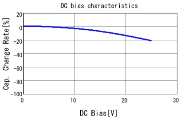
GCJ21BR71E334KA01 C-DC bias capchange, 25.0degC, A
