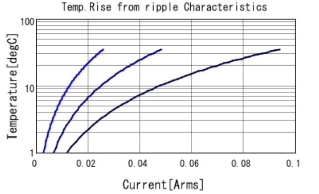
GRM31BR73A681KW01 Temp. rise — 30kHz — 100kHz
