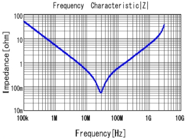
■ GRJ31CR72E333KWJ3 |Z| DCOV, 25degC
