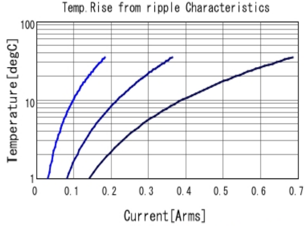
GRJ31CR72E333KWJ3 Temp. rise ■ 30kHz ■ 100kHz ■ 300kHz
